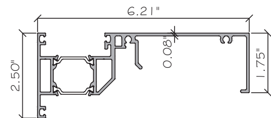
E6 SILL INSIDE ES-W625-G91 ALUM. 6063-T6
