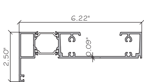
E2 HEAD INSIDE ES-W625-G87 ALUM. 6063-T6
