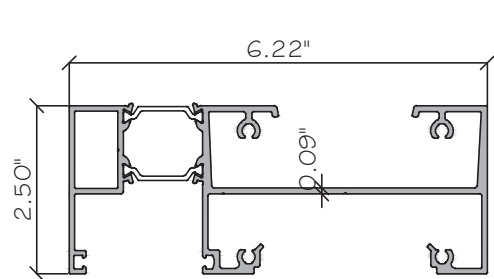
E1 HEAD OUTSIDE ES-W625-G86 ALUM. 6063-T6
