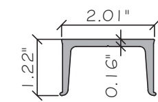
E24 ANCHOR ES-WC25-013 ALUM. 6065-T5
