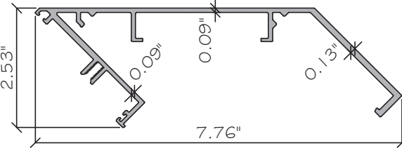
E19 INSIDE CORNER MALE ES-W625-027 ALUM. 6063-T6
