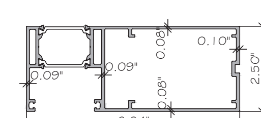
E8 JAMB ES-W625-G93 ALUM. 6063-T6
