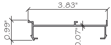
E16 SNAP CLIP ES-W625-017 ALUM. 6063-T5
