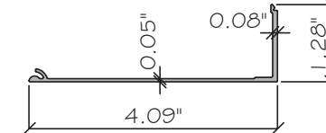
E15 HEAD COVER ES-W625-014 ALUM. 6063-T5
