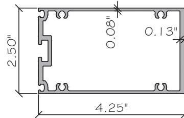
E14 SSG MULLION BACK ES-W625-011 ALUM. 6063-T6
